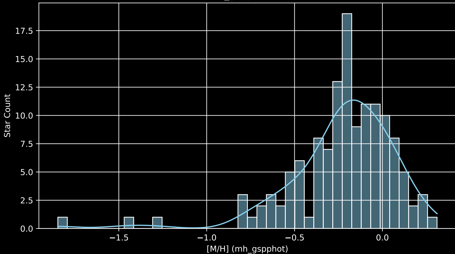
GALAH DR4 Field: [3971] [M/H] (mh_gspphot) (n= 133)
