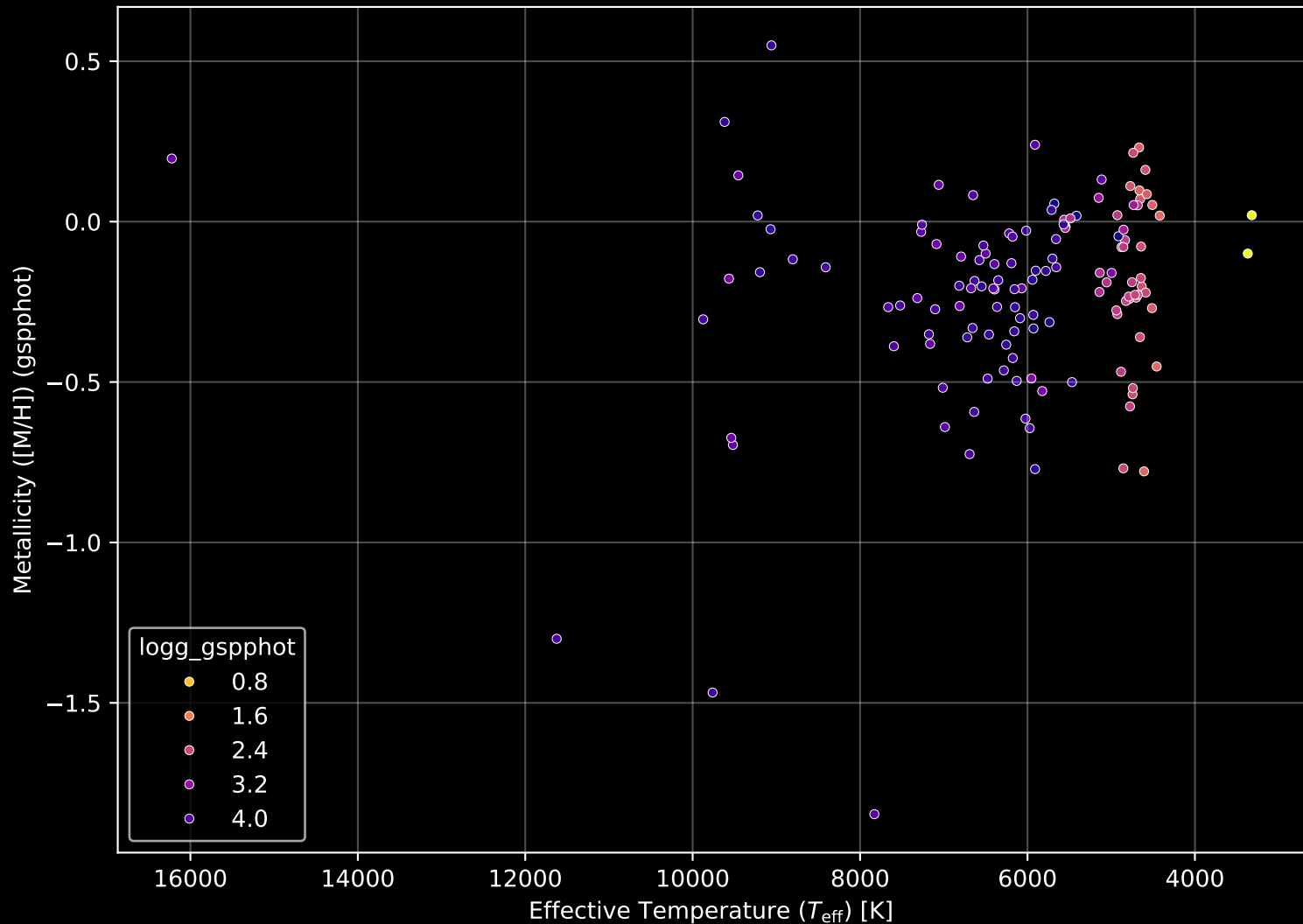
GALAH DR4 Field: [3971] Stellar Population Parameters (n= 134)
