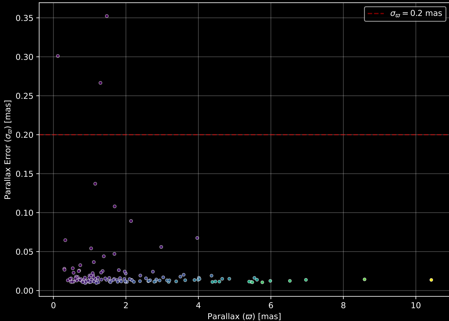
GALAH DR4 Field: [3971] Parallax Quality (n= 134)
