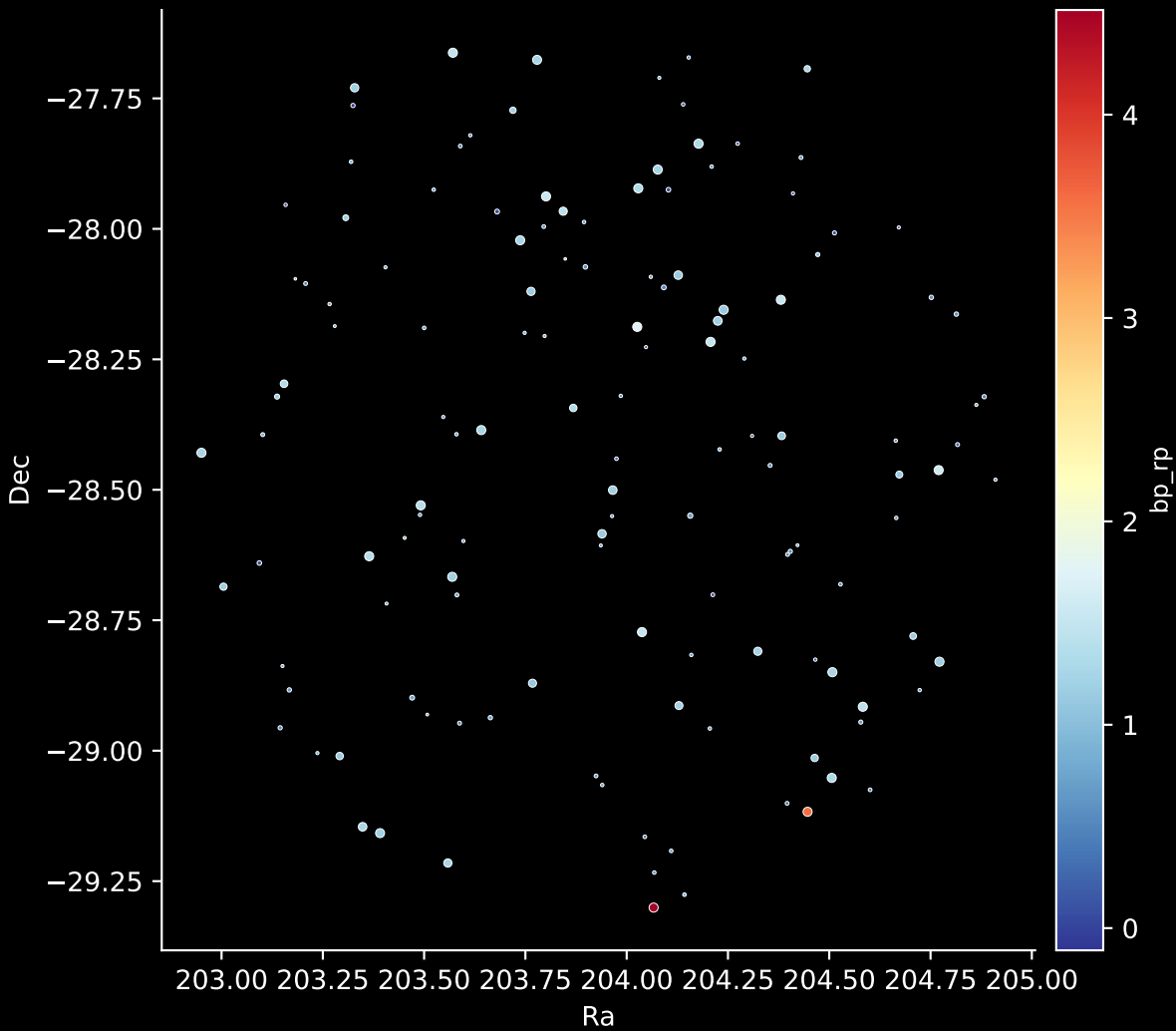
GALAH DR4 Field: [3971] Stars: 134
